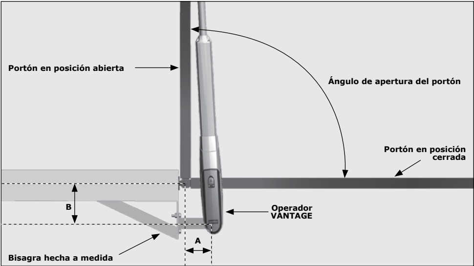
FIGURA 27. VANTAGE 400: PORTÓN DE APERTURA HACIA AFUERA
